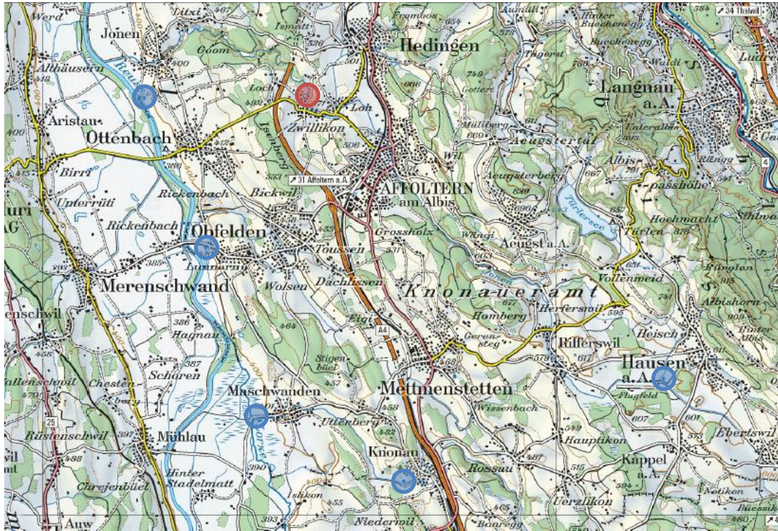
Figur 8: ARA-Standorte im Knonauer Amt (ARA Ottenbach, ARA Affoltern a. A., ARA Obfelden, ARA Maschwanden, ARA Hausen, ARA Knonau, von links oben nach rechts unten). Roter Kreis: prüfenswert; blauer Kreis: nicht prüfenswert.
